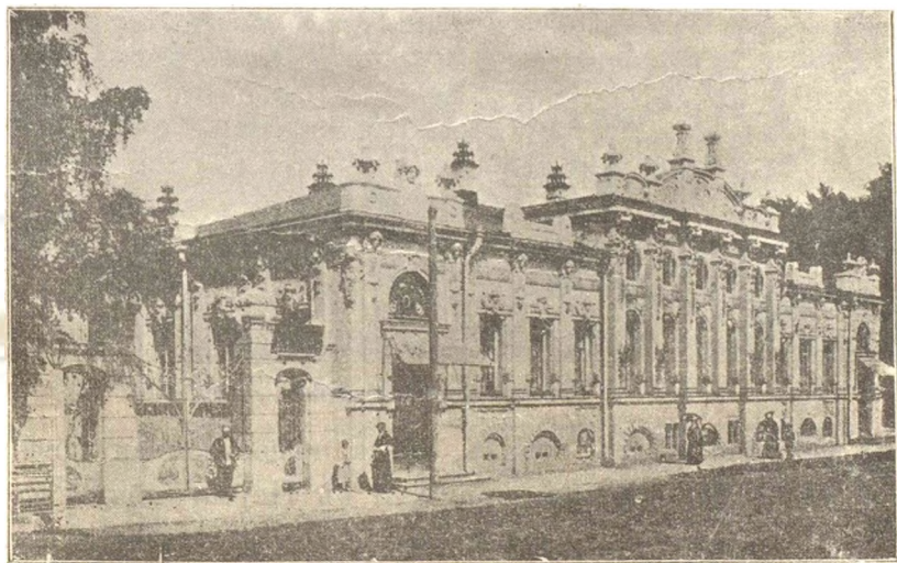
Домъ Грибушина.
