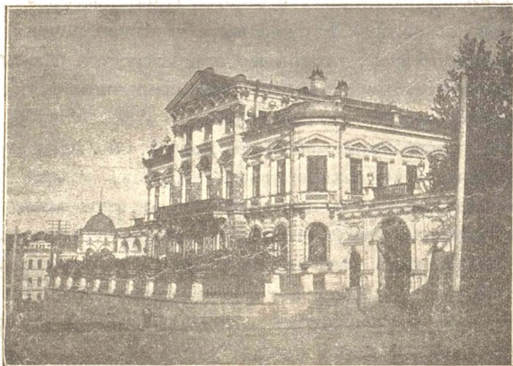
Домъ Мѣшкова.
