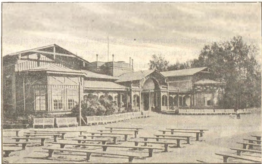
Видъ бульвара.
